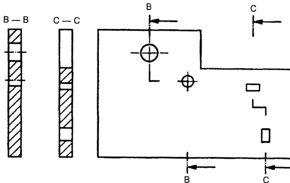
Рисунок 2 — Приклад зображення на машинобудівних кресленнях
